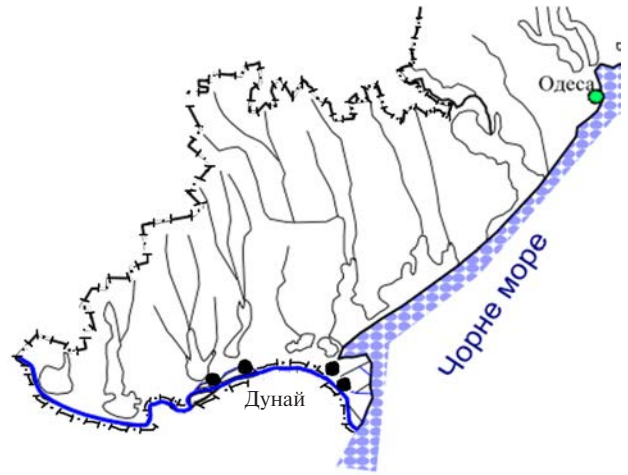
Рис. 2. Картосхема поширення Armoracia macrocarpa на території української частини долини Дунаю (Одеська обл.)
