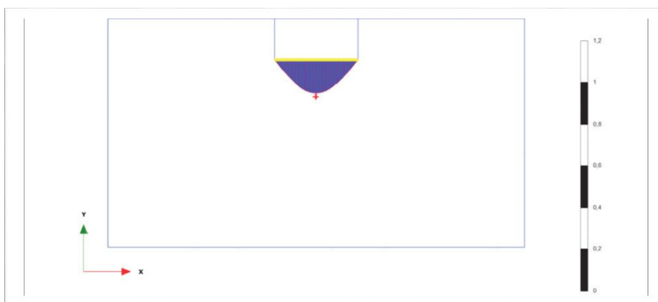
Рис. 11. Епюра зусиль в нижній частині сітки моделі конструкції «ґрунт—геотекстиль» розміром 19.0 × 10.0 см (за даними програмного комплексу PLAXIS)
