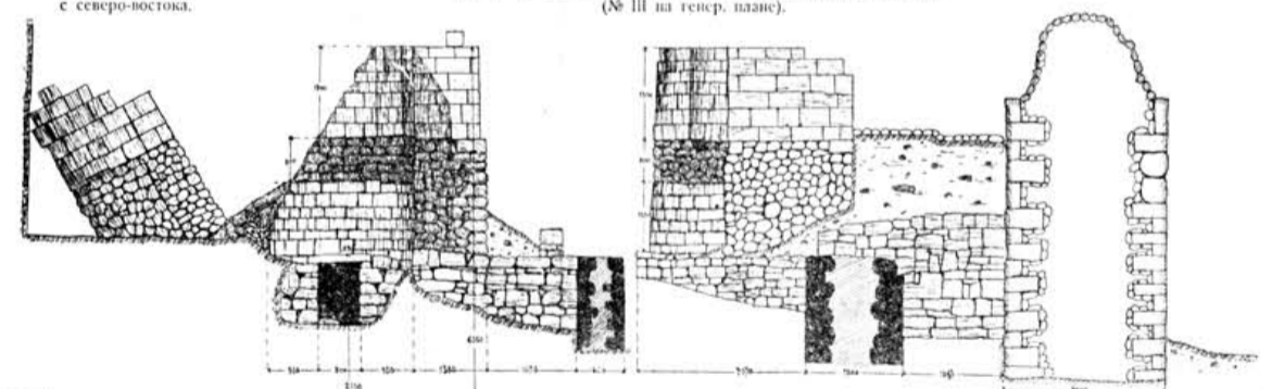
Черт. 9. Чертежи базилика «Асютки, что на забрале».
