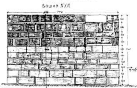
Черт. 6. Развернутый фасад башни № XVI. Нижние 6 рядов — середина IV века до н. эр. Верхние 4 ряда — римской эпохи.
