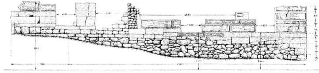
Черт. 5. Древнерусское здание у ворот на 16 куртине («кладовая»).
