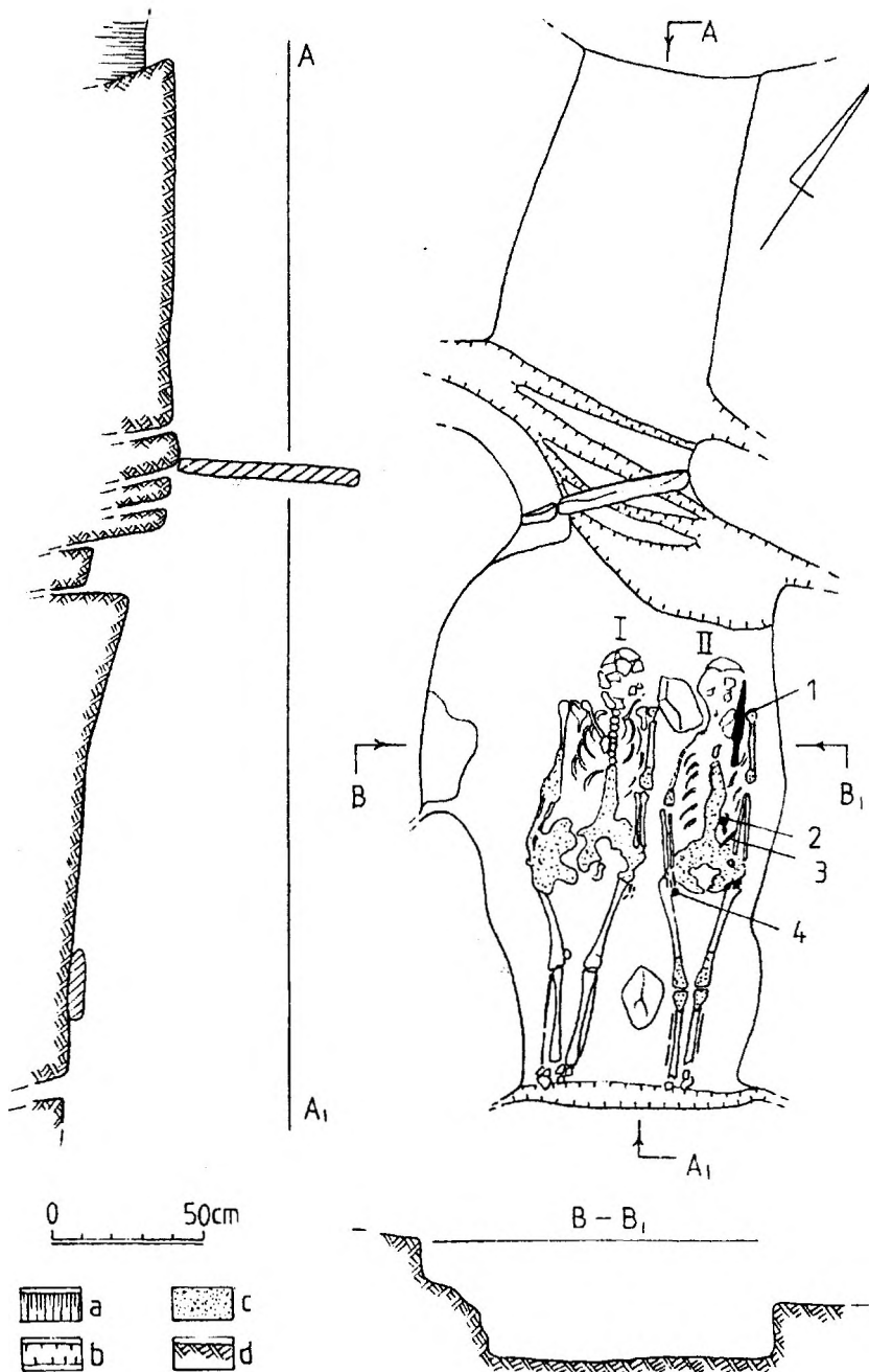
Рис. 9. План и разрезы к плану склепа 109.
