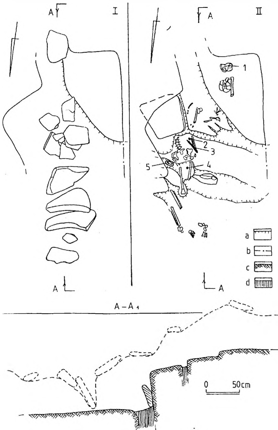
Рис. 2. Могила 91. План и разрез к плану. I – слой с плитами; II – слой с погребением. 1, 5 – лепные сосуды; 2 – бронзовая пряжка; 3 – железный нож; 4 – железная пряжка а – геологические трещины; б – предполагаемые границы могилы; с – материк; d – темный грунт, заполнение трещин.
