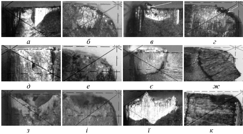
Рис. 6. Характер зношування різальних пластин P1 (а, б, д, е, з, і) і P2 (в, з, є, ж, і, к) при глибині різання 0,2 (а-г), 0,5 (д-ж), 1,0 (з-к) мм.
