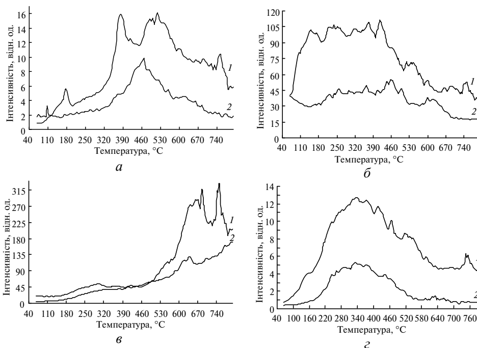
Рис. 3. Інтенсивність термодесорбційних спектрів газів, що виділяються з об'єму різних пластин P1 (1) і P2 (2); m/z = 16 (а), 18 (б), 28 (в), 44 (з).
