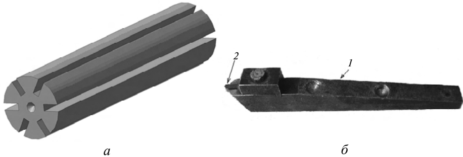
Рис. 2. Заготовка деталі (а) і державка (1) з пластиною (2) в зборі (б) для дослідження зношування та стійкості до ударних навантажень при точінні.
