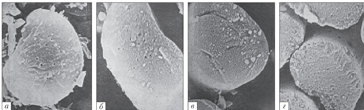
Рис. 1. Мікроструктура вуглецевої волокнистої матриці різного ступеня випалу (%), \times 7500 : a – вихідний; b – 25; c – 41; d – 67
