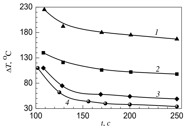
Рис. 3. Зміна в часі обчисленого перепаду температури \Delta T в заготовці при використанні схеми III (із ZrO_2 -диском, рис. 1в) при різній товщині \Delta r стінки графітової прес-форми: 1 – \Delta r = 0,005 м, 2 – \Delta r = 0,010 м, 3 – \Delta r = 0,015 м, висота диску h_d = 0,008 м; 4 – \Delta r = 0,015 м, h_d = 0,012 м
