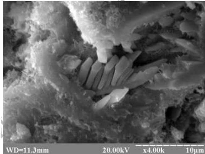
Рис. 1. Мікроструктура каменю КРТМ-ПВ ( \times 4000 ) у середовищі прісної води
