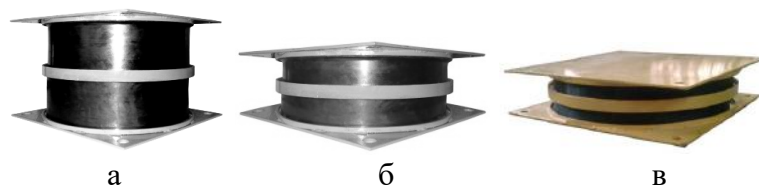
а – сейсмозащитный блок 1-го типа (высота резиновых элементов 2×120 мм, диаметр 400 мм); б – сейсмозащитный блок 2-го типа (высота резиновых элементов 2×70 мм, диаметр 400 мм); в – сейсмозащитный блок 3-го типа (высота резиновых элементов 2×50 мм, диаметром 480 мм и 500 мм)
