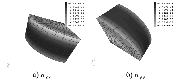
Рисунок 2 – Распределения нормальных напряжений по сейсмоопоре
