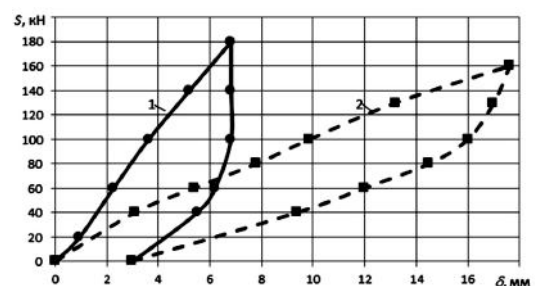
Рисунок 5 – Зависимости «вертикальная нагрузка – перемещение» для ЭБ диаметром 400 мм
