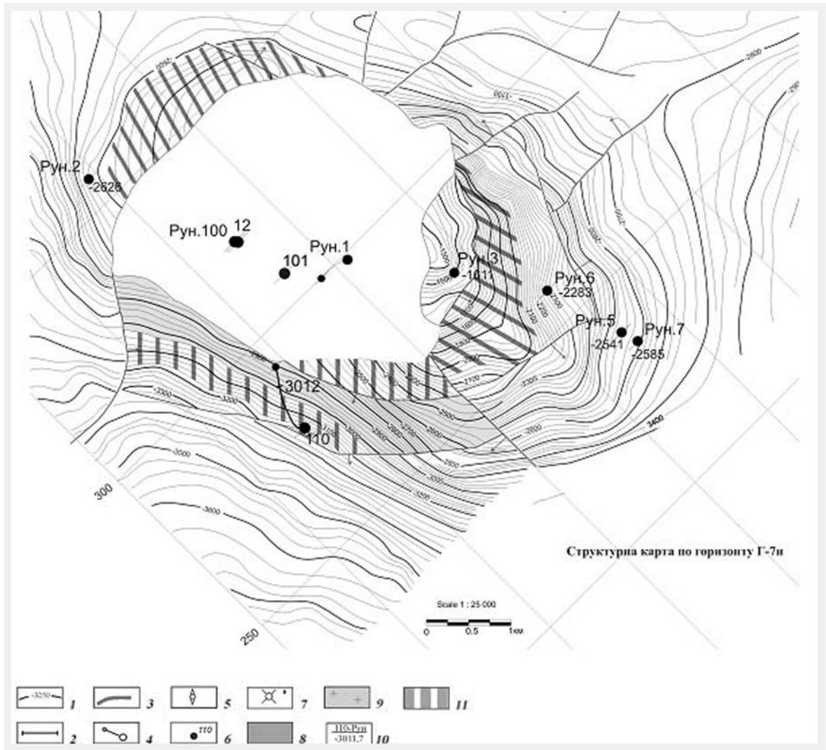
Рис. 2. Структурна карта продуктивного горизонту Г-7н з винесенням контурів встановленої та прогнозованої нафтоносності. Нафтове родовище Академіка Шпака
