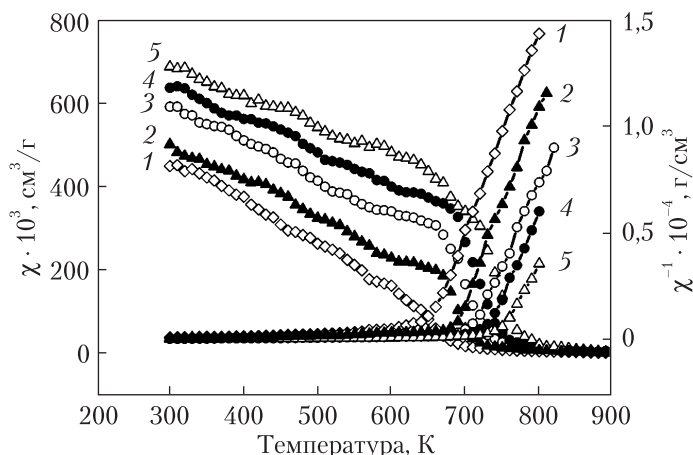
Рис. 1. Графіки прямих \chi(T) та обернених 1/\chi(T) температурних залежностей магнітної сприйнятливості карбиду \text{NiC}_x , отриманого при різній тривалості обробки в кульовому млині: 1 – 150; 2 – 210; 3 – 270; 4 – 315 та 5 – 360 хв
