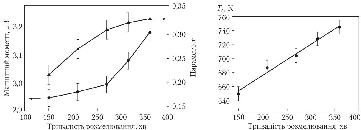
Рис. 2. Залежності ефективного магнітного моменту карбіду \text{NiC}_x та ступеня заповнення його кристалічної ґратки атомами вуглецю від часу обробки шихти в кульовому млині
