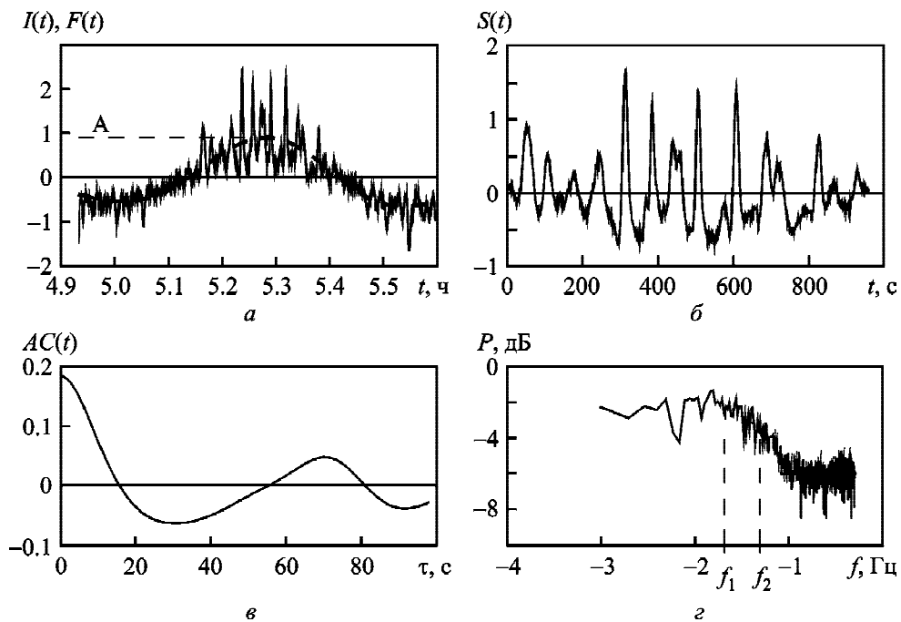
Рис. 1. Пример обработки записи сигнала радиосточника 3C405: a – исходная запись I(t) с вписанной диаграммой направленности F(t) (пунктирная линия); b – мерцания S(t) ; c – автокорреляционная функция мерцаний AC(\tau) ; d – спектр мощности мерцаний P(f) в логарифмической шкале с вписанной прямой линией в выделенном участке в интервале частот 0.02 \div 0.05 Гц
