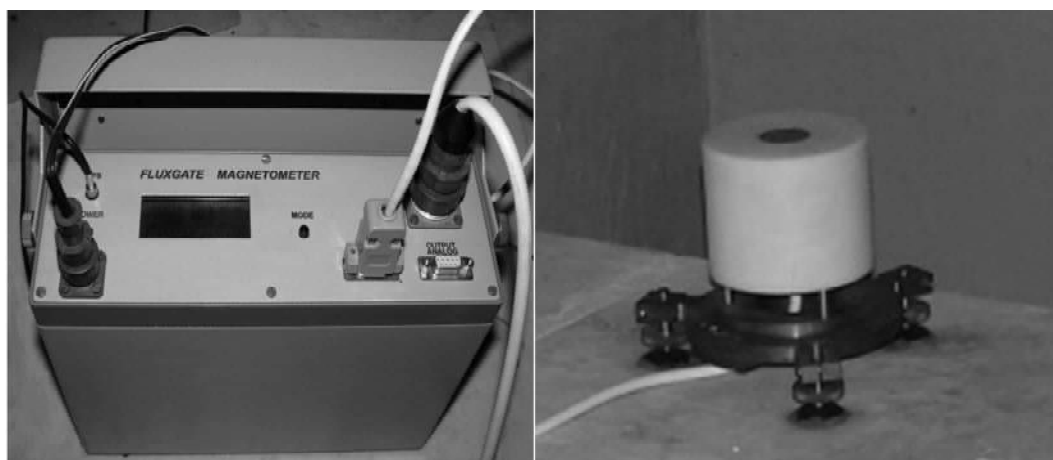
Рис. 2. Общий вид регистрационного блока (слева) и датчика (справа) феррозондового магнитометра LEMI-008
