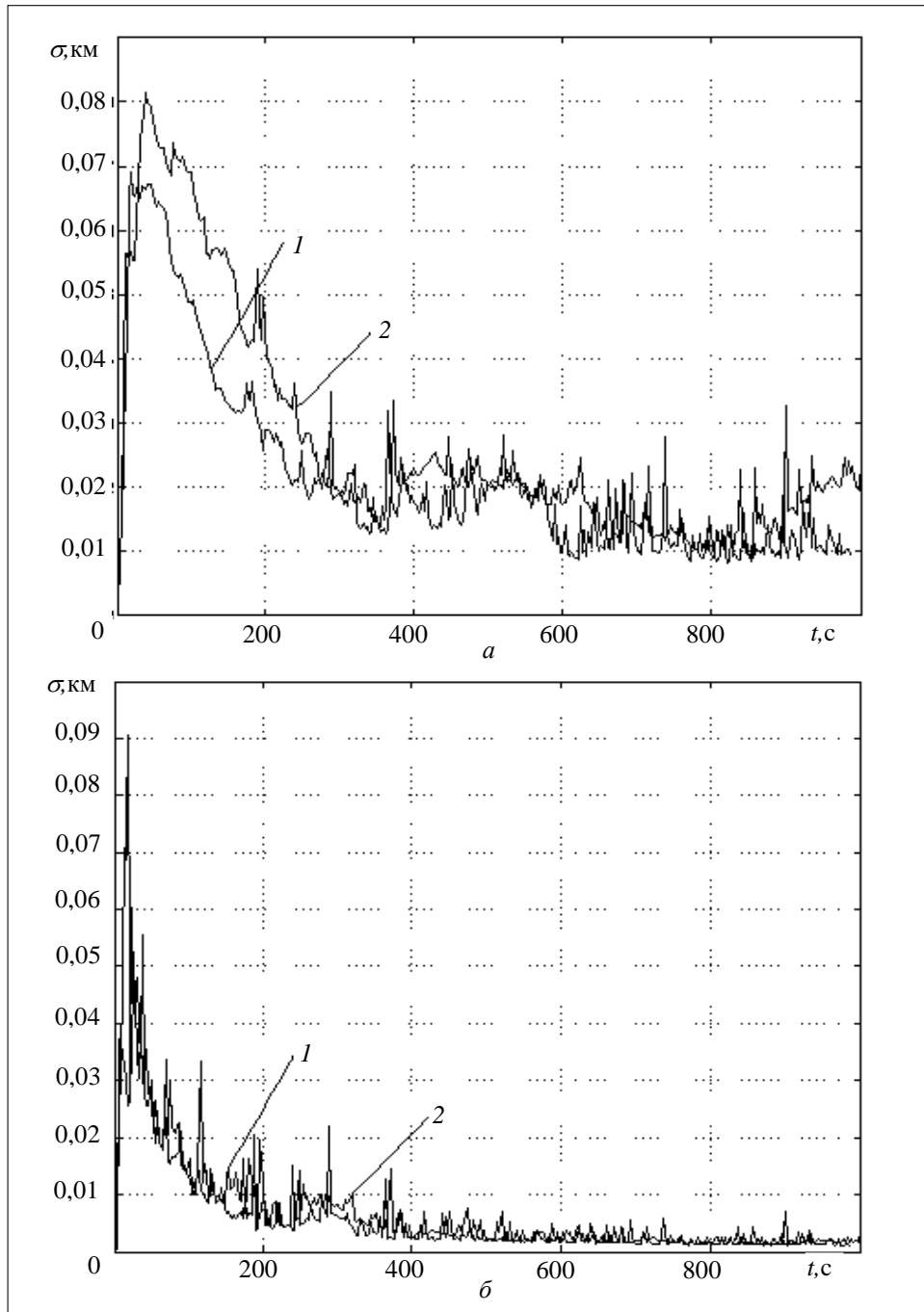
Рис. 2. Среднеквадратические ошибки экстраполяции: а — дальности, б — азимута (1 — адаптивный обобщенный фильтр Калмана; 2 — линейный адаптивный фильтр)
