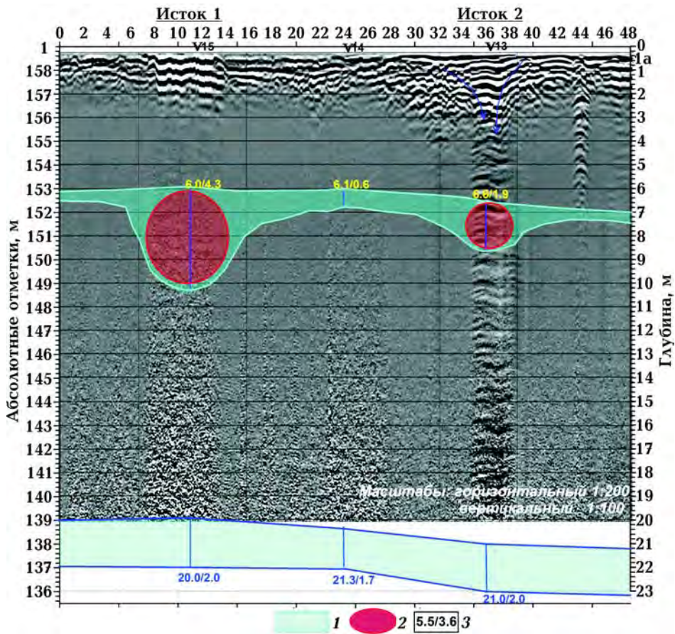
Рис. 9. Вертикальный разрез зоны увлажненных грунтов на строительном участке жилого комплекса по ул. В. Липковского 37г в Соломенском районе г. Киева. Профиль 1: 1 — зона повышенного увлажнения почв; 2 — зоны повышенной фильтрации грунтовых вод (техногенные водные потоки); 3 — 5,5/3,6 — глубина до водного горизонта/мощность.
