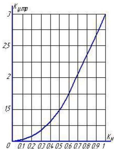
Рис. 3 Зависимость кратности увеличения потерь активной мощности в трансформаторе от коэффициента неравномерности
