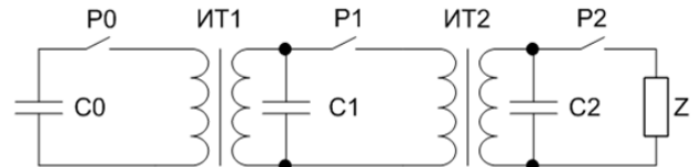
Рис. 1. Схема генератора
