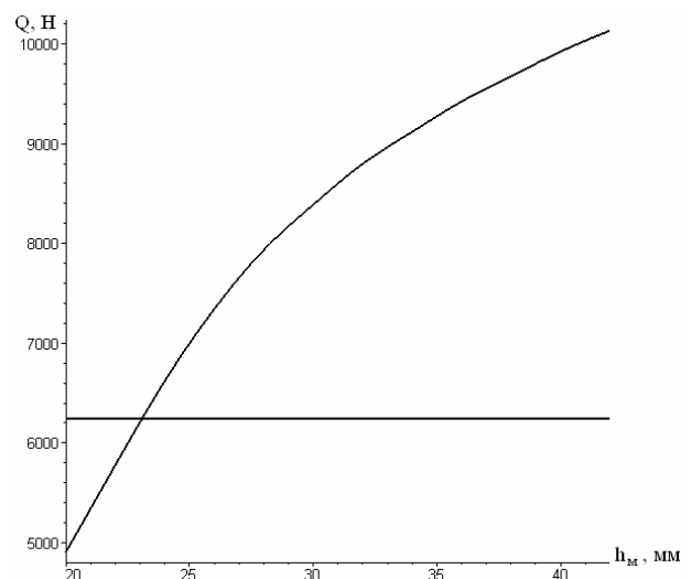
Рис. 4. Зависимость удерживающего тягового усилия от высоты постоянного магнита и противодействующая сила выключателя
