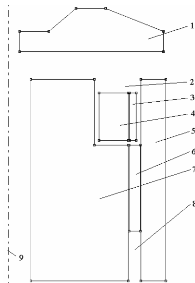
Рис. 3. Расчетная модель магнитной системы электромагнита с однопозиционной магнитной защелкой (1 - якорь, 2 - пространство для установки катушки, 3 - отключающая обмотка, 4 - включающая обмотка, 5 - корпус, 6 - постоянные магниты, 7 - сердечник, 8 - воздушный зазор (шунт), 9 - ось симметрии магнитной системы)
