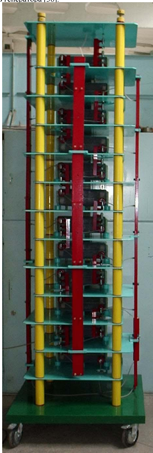
Рис. 7. Общий вид передвижного ГИН на номинальное напряжение 1,2 МВ с запасаемой энергией в 15 кДж
