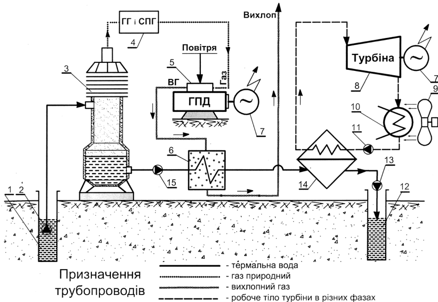
Рис. 4. Схема комбінованої електрогенеруючої установки з передачею скидної теплоти ГД в теплообмінник ГЭС.
