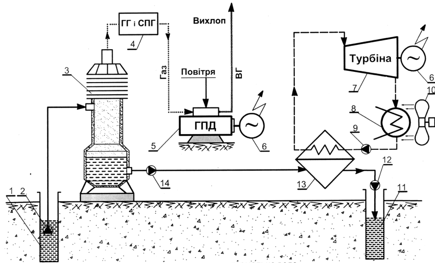
Рис. 3. Схема комбінованої електрогенеруючої установки на ГЭС, теплоносій якої насичений природним газом, з вихлопом ГД у атмосферу.
