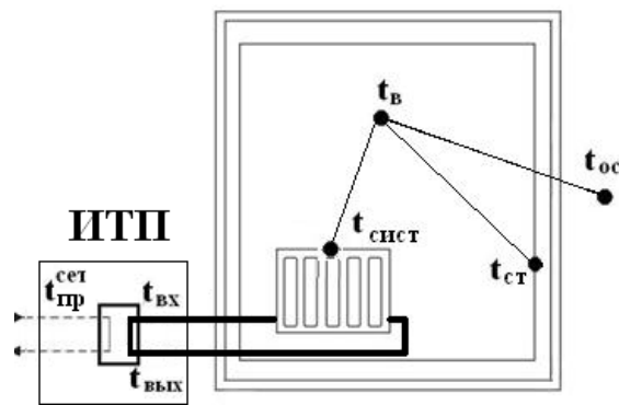
Рис. 1. Схема рассматриваемого здания с указанием узлов и тепловых связей модели.
