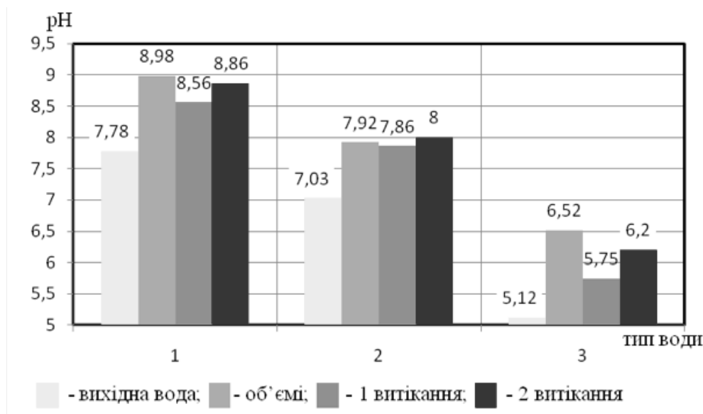
Рис. 2. Зміна водневого показника в залежності від способу організації процесу скидання тиску ( P = 10 кПа, \Delta T = 15 °С): 1 – водопровідна вода, 2 – артезіанська вода, 3 – дистильована вода.
