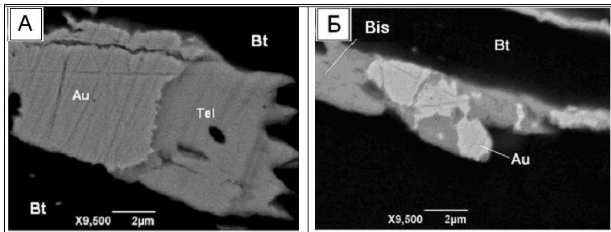
Рис. 2. Мікросрастання самородного золота з теллуридом висмута (А) і висмутином (Б). Аншлиф. Електронні знімки. Скв. 3052, гл. 213,3 м.
