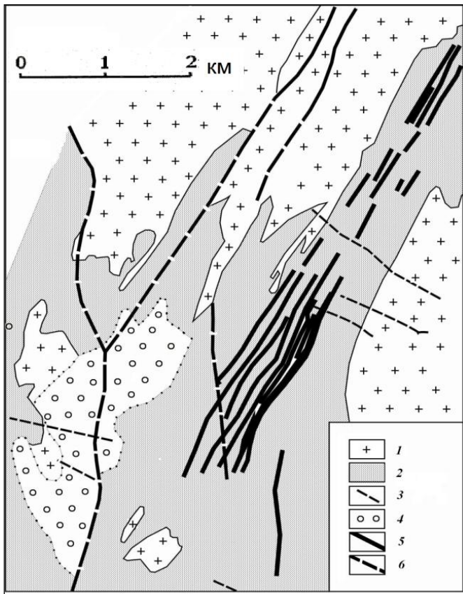
Рис. 1. Геолого-структурная схема Юрьевского рудного поля (по данным КП «Кировгеология») 1 – гранитоиды кировоградского комплекса;
