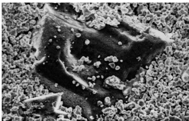
Рис.2. Фрагмент рабочей поверхности диска с единственным зерном алмаза (×2000)
