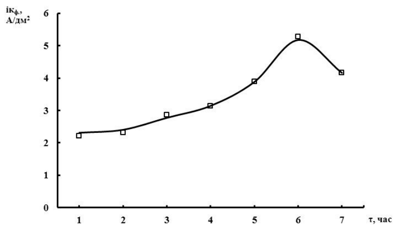
Рис. 1. Зависимость фактической плотности тока i_{кф} , А/дм 2 , от продолжительности зарачивания зерен марки АС20 зернистостью 400/315
