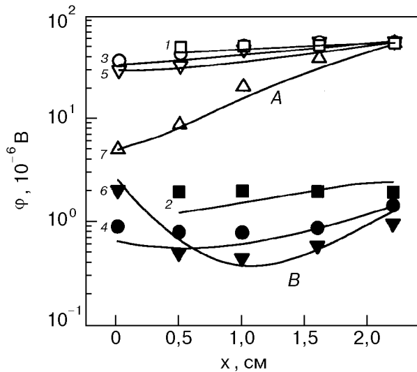
Рис. 5. Потенциал \phi как функция координаты вдоль потока заряда на боковых гранях (A — грань образца, соответствующая сильному сигналу, B — слабому) при различных параметрах неоднородности k , Тл/см; \alpha , Тл/см 2 : 0,9; 0,1 (1, 2); 1,0; 0,5 (3, 4); 0,7; 1,0 (5, 6); 0,15; 2,6 (7). Символы — эксперимент, линии — теория.
