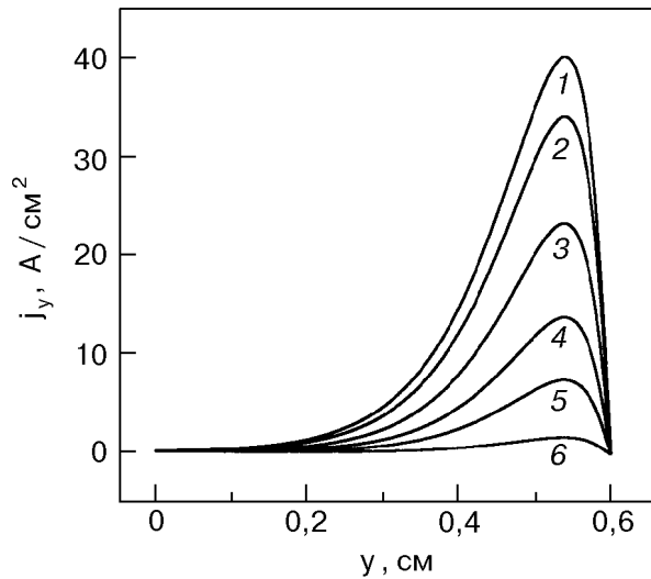
Рис. 3. Теоретическая зависимость плотности поперечного тока j_y от координаты y при некоторых значениях параметра неоднородности (6) f(x) , \text{см}^{-1} : 15,7 (1); 16,0 (2); 16,3 (3); 16,5 (4); 16,6 (5); 16,7 (6).
