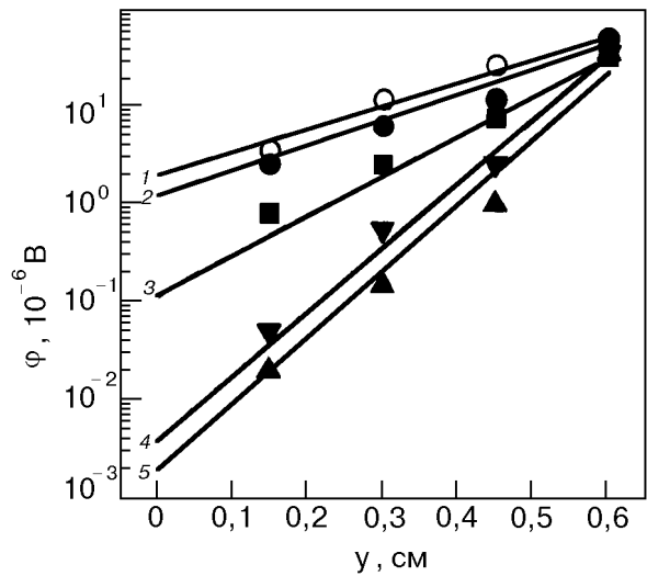
Рис. 6. Зависимости потенциала \phi от поперечной координаты для ряда значений параметров неоднородности k , Тл/см; \alpha , Тл/см 2 : 0,9; 0,1 (1, 2); 0,7; 1,0 (3); 1,0; 0,5 (4); 0,15; 2,6 (5) при различных величинах локального магнитного поля B , Тл: 6,75 (1); 5,8 (2); 4,34 (3); 4,73 (4); 3,09 (5). Символы — эксперимент, линии — теория.
