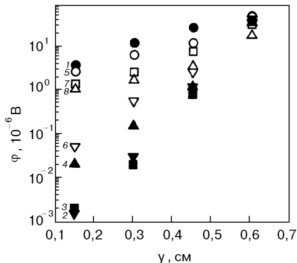
Рис. 1. Зависимость потенциала \varphi от координаты в направлении, нормальном транспорту заряда, для экспоненциального типа неоднородности при различных значениях относительного градиента d , \text{см}^{-1} : 0,1 (1, 5); 0,4 (2, 6); 0,6 (3, 7); 1,1 (4, 8) и локального магнитного поля B , Тл: 6,85 (1); 6,50 (5); 6,0 (2); 5,35 (3); 5,20 (6); 4,20 (7); 3,95 (4); 2,40 (8).
