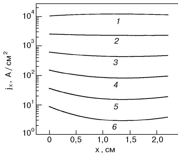
Рис. 4. Аналитическое распределение плотности тока j_x вдоль градиента поля при различных значениях поперечной координаты y , см: 0,6 (1); 0,5 (2); 0,4 (3); 0,3 (4); 0,2 (5); 0,1 (6).
