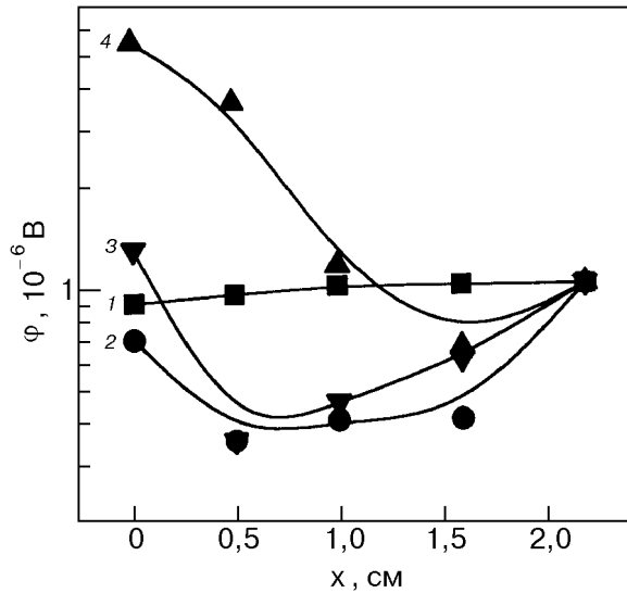
Рис. 2. Распределение потенциала \phi вдоль потока заряда на боковой грани образца, соответствующей слабому сигналу, при различных уровнях градиентности магнитного поля d , \text{см}^{-1} : 0,1 (1); 0,4 (2); 0,6 (3); 1,1 (4).
