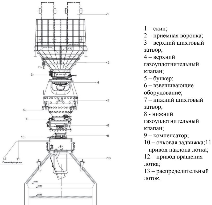
Рис. 1. Схема бесконусного загрузочного устройства ДП №3 ПАО «ЕМЗ».
