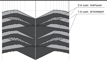
Рис.7. Расчетная структура столба шихты на колошнике после выгрузки цикла загрузки, в котором две порции ЖРМ выгружаются поскипово
