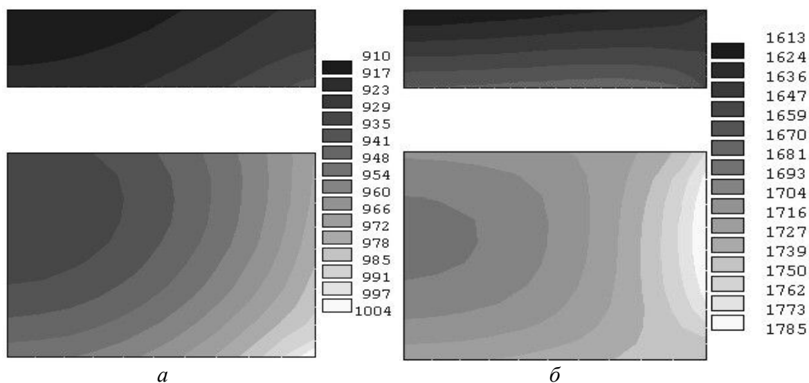
Рис. 6. Розподіл температури (К) в інфільтраті та SiC-заготовці в різні моменти часу: а – 2400 с; б – 5717 с (висота індуктора – 0,6 м)
