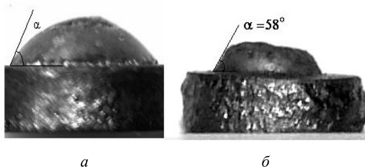
Рис. 3. Загальний вигляд крапель розплавів Со–W (а) та Си–Ті (б) на поверхні нанокompозиту алмаз – карбід вольфраму (а) та полікристалу, спеченого з алмазного порошку марки АСМ 1/0 (б)
