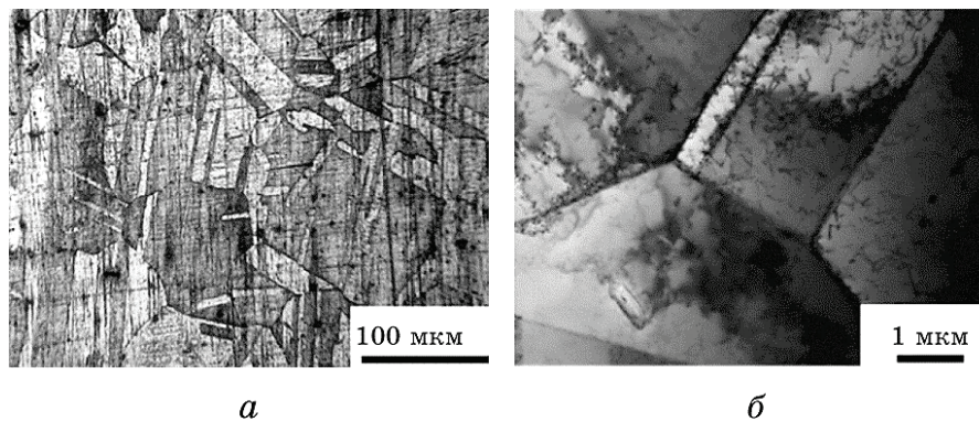
Рис. 2. Оптичне ( a ) і ТЕМ зображення ( б ) мікроструктури аустенітної сталі у вихідному стані.
