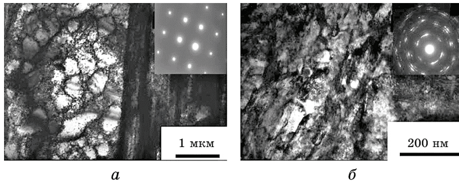
Рис. 11. TEM-зображення мікроструктури та відповідні картини електронної дифракції неіржавійної сталі 12Х18Н10Т після УЗУО в середовищі газу аргону ( a ) та рідкого азоту ( б ) впродовж 250 с.
