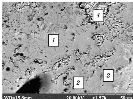
Рис. 4. Мікроструктура та хемічний склад різних областей поверхні неіржавійної сталі 12X18Ni10Ti після УЗУО ( A = 25 \text{ мкм} ) впродовж 150 с на повітрі ( a ) та в середовищах газу аргону ( б ) і рідкого азоту ( в ).
