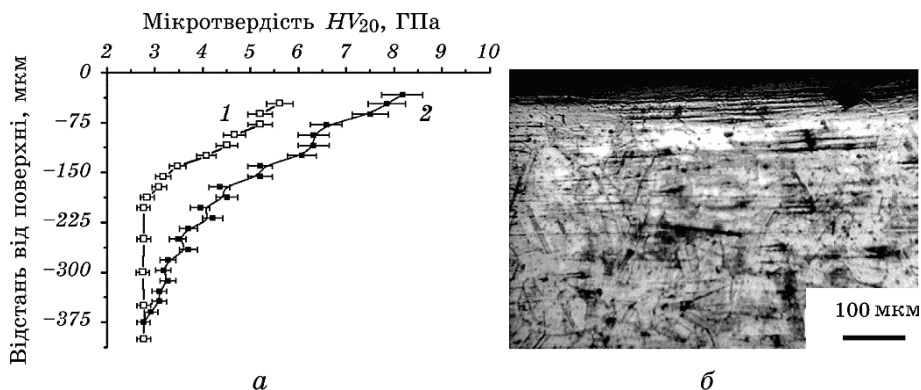
Рис. 9. Розподіл мікротвердості (а) та оптичне зображення мікроструктури (б) у поперечному перерізі зразка сталі 12X18N10T після УЗУО в середовищі рідкого азоту впродовж 150 с (б, 1) та 250 с (2).
