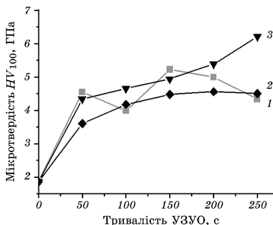
Рис. 3. Зміна мікротвердості поверхні зразків неіржавійної сталі після УЗУО в різних середовищах ( A = 25 \text{ мкм} ): 1 — повітря, 2 — аргон, 3 — рідкий азот.
