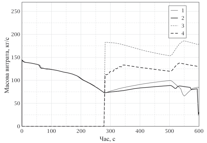
Рис. 2. Масові витрати для течі Ду 40 мм: 1 — витрата в течу за базовим варіантом; 2 — витрата в течу з ПК САОЗ ВТ; 3 — витрата від САОЗ ВТ за базовим варіантом; 4 — витрата від САОЗ ВТ з ПК
