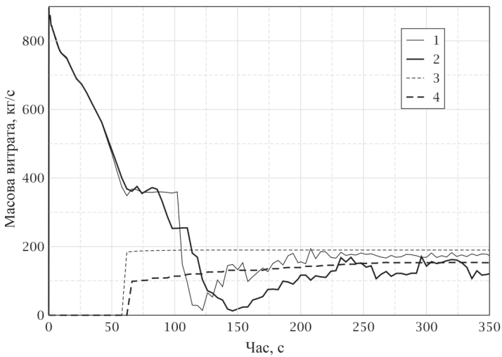
Рис. 3. Масові витрати для течі Ду 100 мм: 1 — витрата в течу за базовим варіантом; 2 — витрата в течу з ПК САОЗ ВТ; 3 — витрата від САОЗ ВТ за базовим варіантом; 4 — витрата від САОЗ ВТ з ПК
