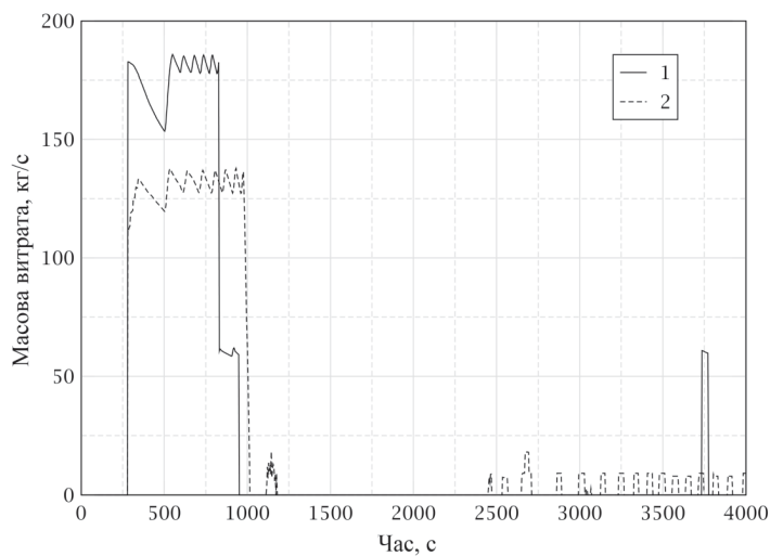
Рис. 5. Масова витрата від насосів САОЗ ВТ (сценарій без додаткових відмов): 1 — базовий варіант; 2 — з ПК САОЗ ВТ
