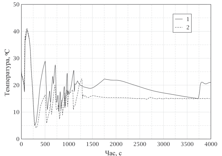
Рис. 6. Мінімальний запас до температури насичення в гарячих нитках ГЦТ (сценарій без додаткових відмов): 1 — базовий варіант; 2 — з ПК САОЗ ВТ
