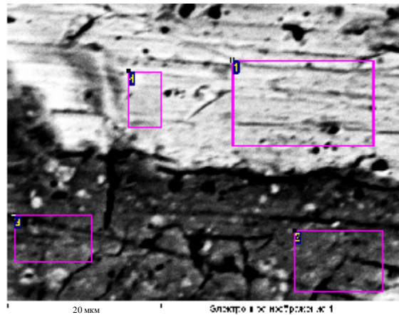
Рис. 7. Мікроструктура та розподіл хімічних елементів (% (мас.)) в пантографічних накладках НМГ-1200 виробництва НТЦ "Реактивелектрон" після експлуатаційних випробувань.
