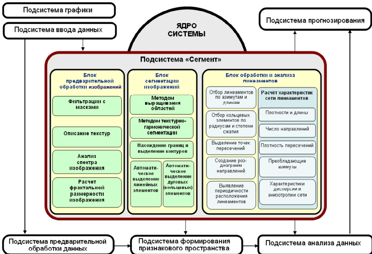
Рис. 4. Функциональная схема подсистемы «Сегмент»
