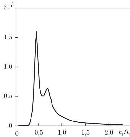
Рис. 4. Трансформований спектр
