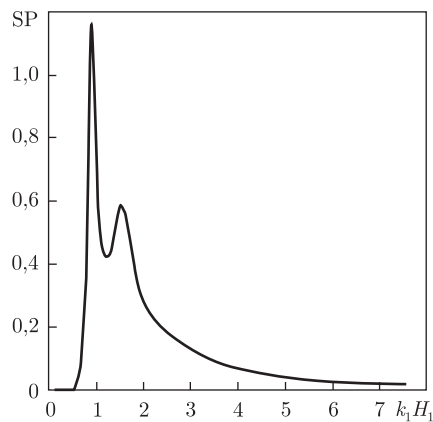
Рис. 3. Двопіковий спектр
