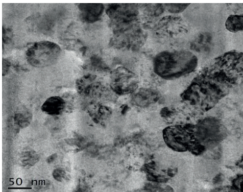
Рис. 4. Нанокерамика на основе нитрида титана, полученная в ЭРС режимах, разработанных в ИПМ НАН Украины им. И. Н. Францевича [5]
