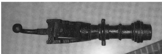
Рис. 3. Стволы орудий, подобные «крымскому» образцу.
