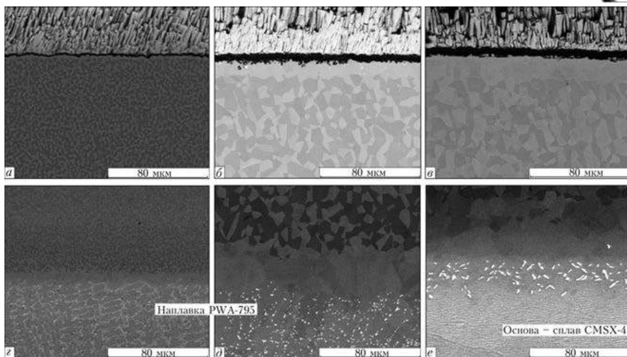
Рис. 7. Состояние межфазных границ связующий слой/керамика (а-в) и основа/связующий слой (з-е) до (а, з) и после (б, в, д, е) испытаний
