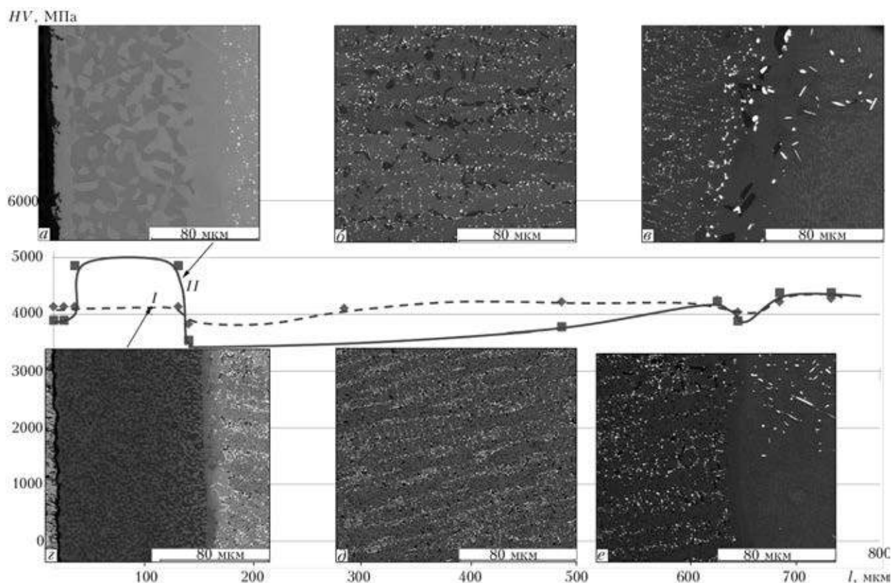
Рис. 5. Микротвердость основных зон ТЗП на наплавленном металле после 300 ч термоциклических испытаний (а–в, II) и до них (г–е, I)
