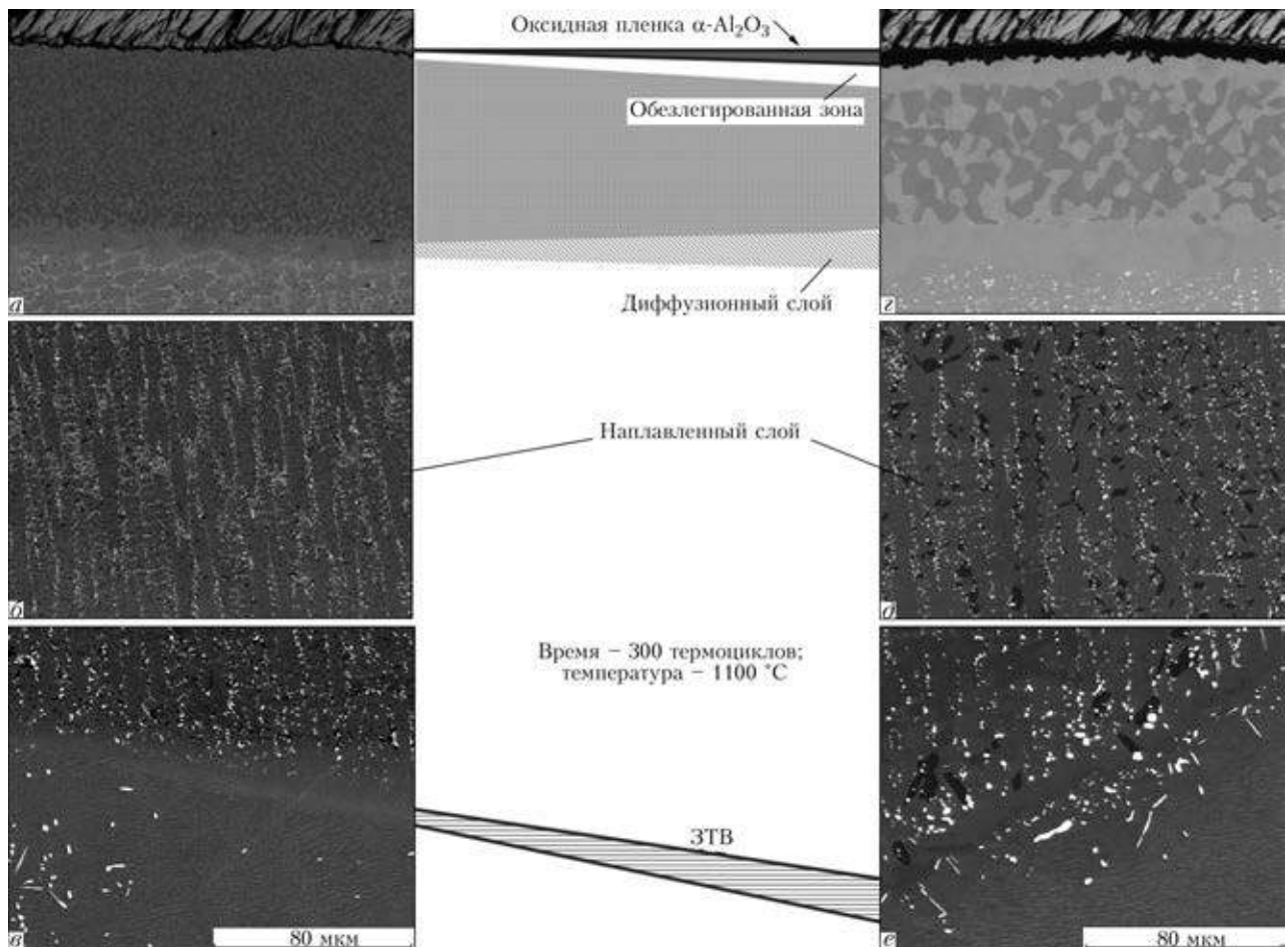
Рис. 4. Эволюция основных зон ТЗП (а-е) при термоциклических испытаниях
