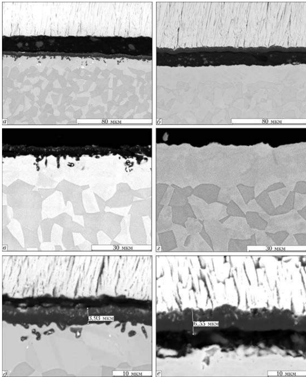
Рис. 8. Адгезия и структура TGO на металлическом подслое после 300 термоциклов испытаний на наплавленном материале (а, в, д) и материале основы (б, з, е)
