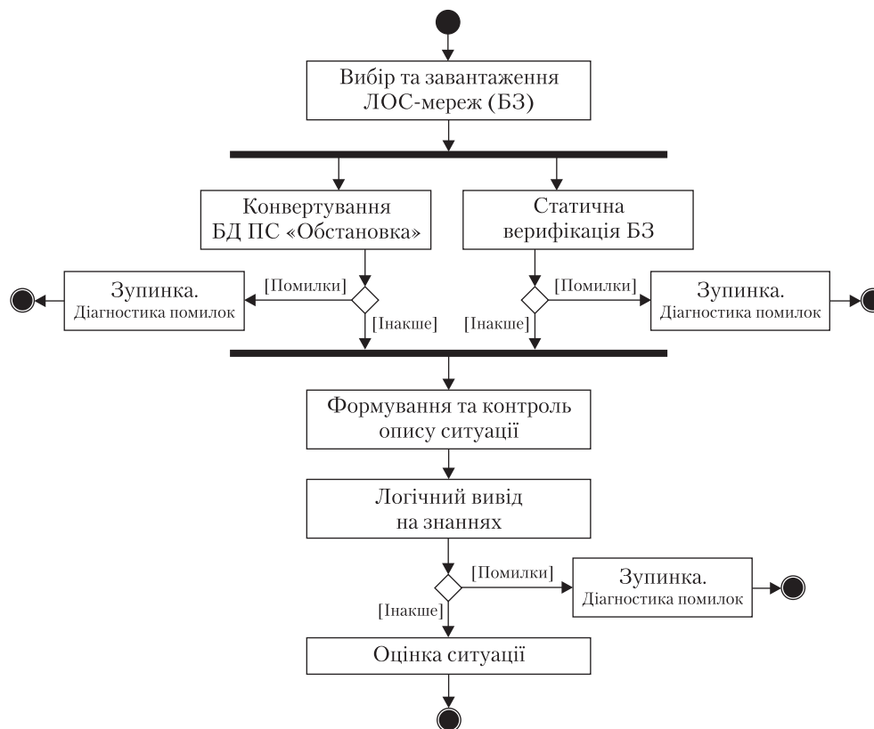
Рис. 5. Діаграма діяльності щодо оцінки ситуації
