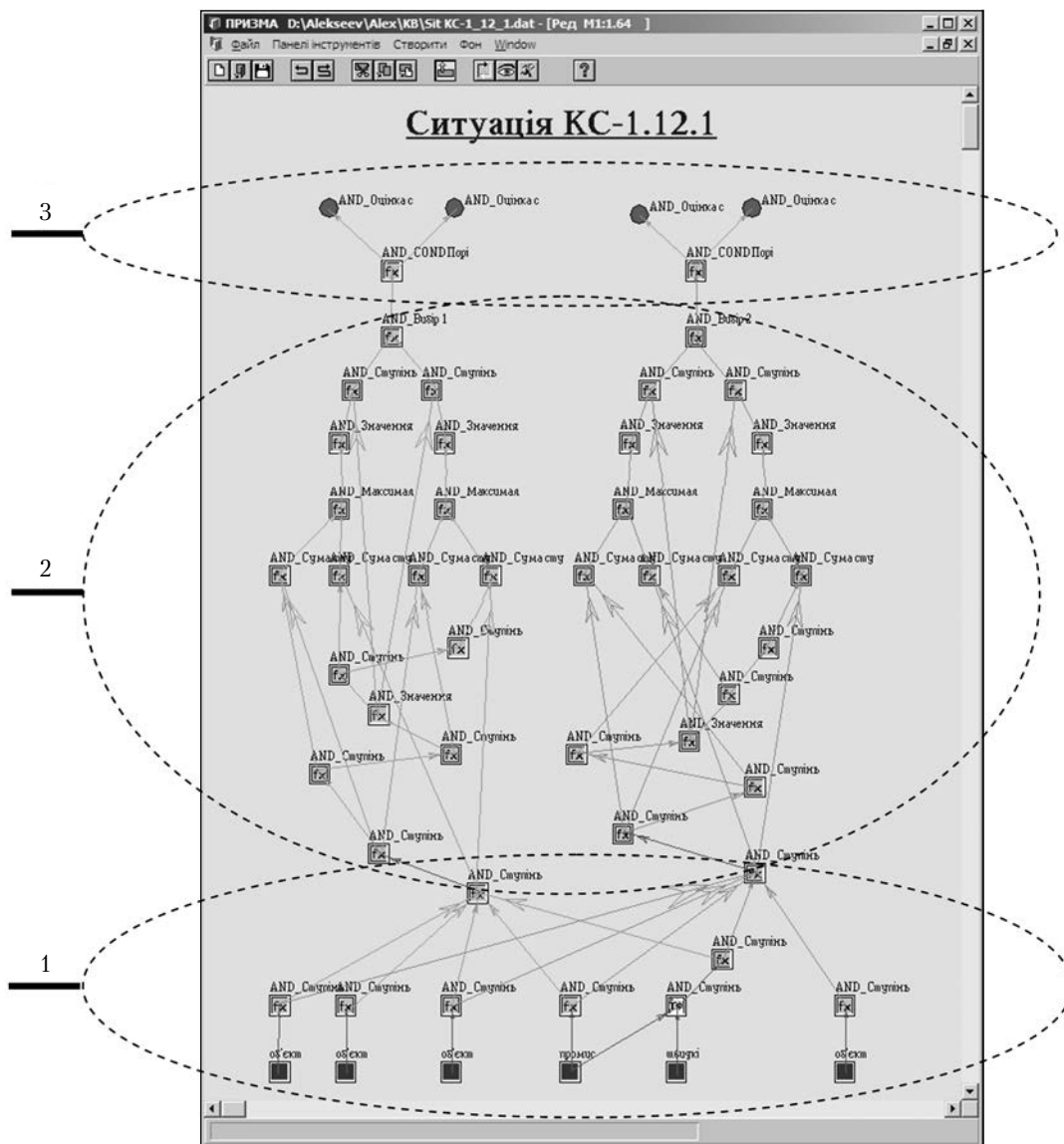
Рис. 3. ЛОС-мережа, в якій подані нечіткі знання про оцінку ситуації
