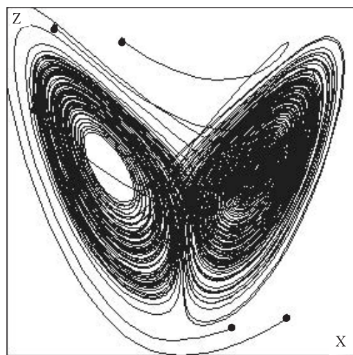
Рис. 4. Утворення дивного атратора Лоренца з різних точок фазового простору за умови t = 30 у.о.
