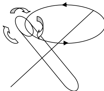
Рис. 7. Протонная прецессия
