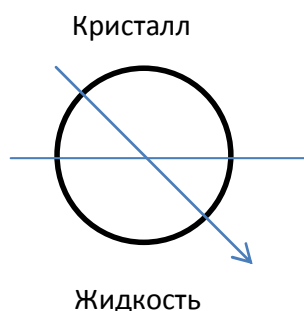
Рис. 3. Проникновение фотона из кристалла в жидкость под углом
