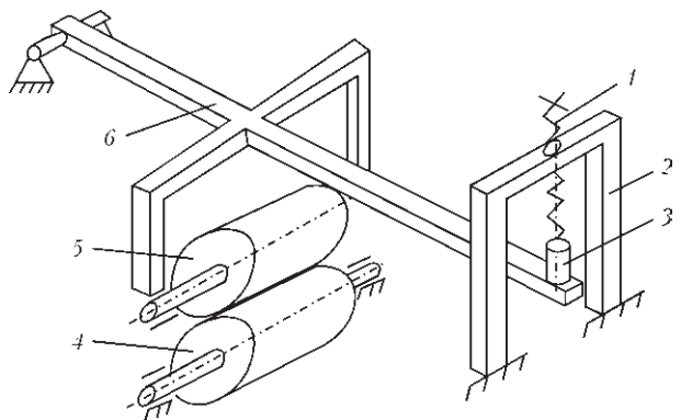
Рис. 3. Кинематическая схема тянущей клетки: 1 — винт; 2 — неподвижная опора; 3 — датчик давления; 4 — неподвижный валок; 5 — верхний подвижный валок; 6 — рычаг; 7 — ось
