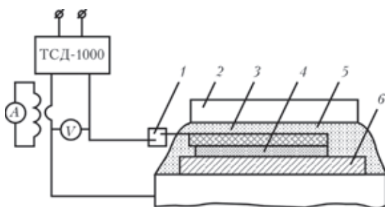
Рис. 1. Наплавка лежачим пластинчатым электродом по слою легирующей присадки: 1 — токоподвод; 2 — медная плита; 3 — электрод; 4 — легирующая присадка; 5 — флюс; 6 — изделие
