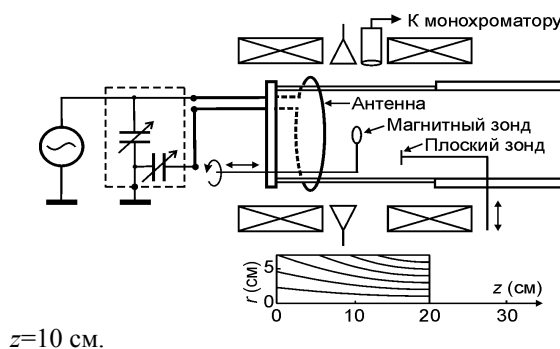
Рис.1. Схема экспериментальной установки (вверху) и профиль силовых линий в неоднородном поле (внизу)
