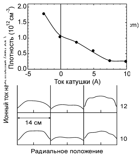
Рис. 4. Плотность плазмы ( z = 10 см) в зависимости от тока левой катушки
