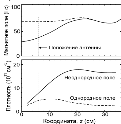
Рис. 2. Продольные профили магнитного поля и плотности плазмы на оси
