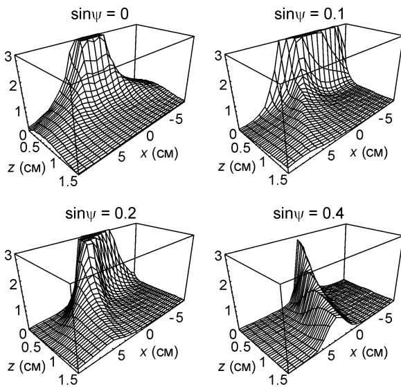
Рис.13. Профили поглощенной мощности при различных наклонах магнитных линий (в \text{mWt}\cdot\text{cm}^{-3}\cdot\text{A}^{-2} ). Параметры вычислений те же, что на рис.12
