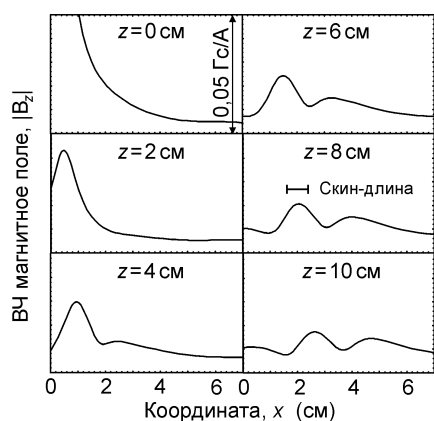
Рис.16. Профили амплитуды магнитного поля. Профили амплитуды ВЧ магнитного поля B_z вдоль координаты x приведены на рис.16 при разных значениях z . При z > 4 см на профиле видны два пика, движущиеся внутрь плазмы, причем траектория минимума между ними идет практически вдоль силовой линии. Эти пики соответствуют резонансным конусам, которые в данном случае проявляются намного отчетливее, чем на профилях поглощения, и весьма похожи на наблюдаемые (ср. рис.5).
