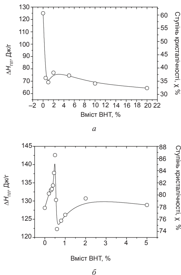
Рис. 2. Залежність ентальпії плавлення та ступені кристалічності від вмісту ВНТ для нанокompозитів на основі ПП (а) та ПЕО (б)
