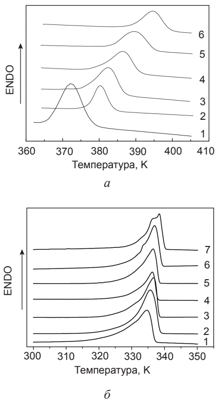
Рис. 1а: ендотерми плавлення для ПП (1) і нанокompозитів на основі ПП, які містять ВНТ: 1 % — 2; 2 % — 3; 5 % — 4; 10 % — 5; 20 % — 6; б: ендотерми плавлення для ПЕО (1) і нанокompозитів на основі ПЕО, які містять ВНТ: 0,2 % — 2; 0,4 % — 3; 0,6 % — 4; 0,8 % — 5; 1 % — 6; 2 % — 7
