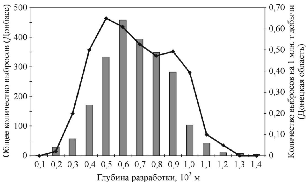
Рис. 1. Изменение общего и удельного (на 1 млн. т добычи) количества внезапных выбросов в зависимости от глубины ведения горных работ в Донбассе и по Донецкой области соответственно: \blacksquare — общее количество выбросов (Донбасс), \blacklozenge — количество выбросов на 1 млн. т добычи (Донецкая область)
