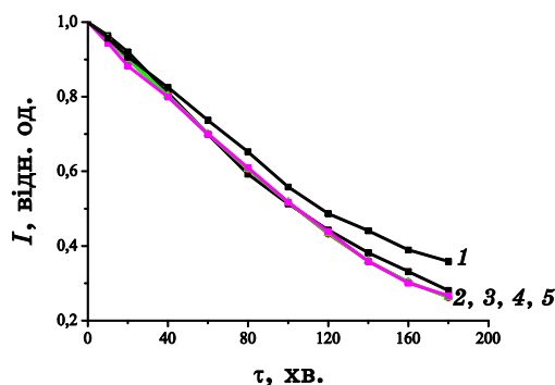
Рис. 7. Кінетичні криві фотовідновлення біхромату калію в присутності EDTA 1:1 на плівках \text{TiO}_2/\text{ZrO}_2/\text{SiO}_2 , опромінені пучком електронів з E = 1,9 МеВ та різними дозами: 1 — неопромінений, 2 — 0,5 МГр, 3 — 1 МГр, 4 — 2 МГр, 5 — 4 МГр. 8
