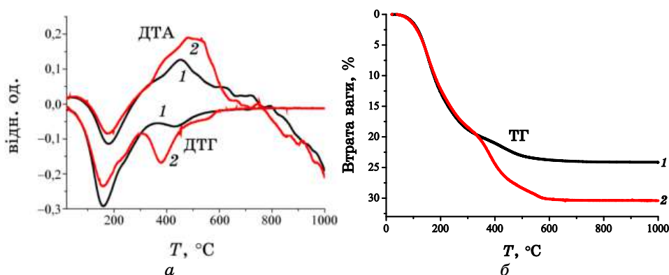
Рис. 3. a — термограми порошоків: \text{TiO}_2/\text{ZrO}_2/\text{SiO}_2 (30%) (1) та \text{TiO}_2/\text{ZrO}_2/\text{SiO}_2 (70%) (2); б — термогравіметричні криві порошоків \text{TiO}_2/\text{ZrO}_2/\text{SiO}_2 з різним вмістом \text{SiO}_2 : 30 ваг.% (1), 70 ваг.% (2). 4
