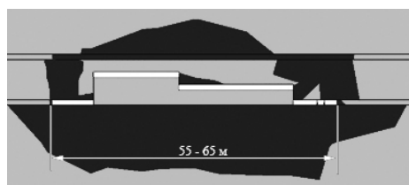
Рис. 3. Распределение зон предельного состояния горных пород при отходе лавы до 55 – 65 м: ■ область действия допустимых напряжений; ■ область предельного состояния
