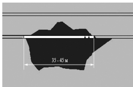
Рис. 2. Распределение зон предельного состояния горных пород при отходе лавы до 35 – 45 м: ■ область действия допустимых напряжений; ■ область предельного состояния
