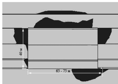
Рис. 4. Распределение зон предельного состояния горных пород при отходе лавы до 65 – 75 м: ■ область действия допустимых напряжений; ■ область предельного состояния
