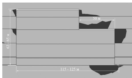
Рис. 7. Распределение зон предельного состояния горных пород при отходе лавы до 105 – 115 м: ■ область действия допустимых напряжений; ■ область предельного состояния
