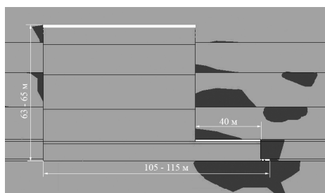
Рис. 6. Распределение зон предельного состояния горных пород при отходе лавы до 105 – 115 м: ■ область действия допустимых напряжений; ■ область предельного состояния
