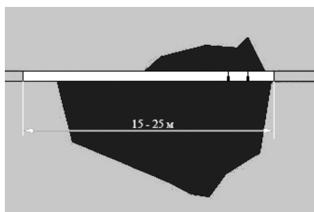
Рис. 1. Распределение зон предельного состояния горных пород при отходе лавы до 25 м: ■ область действия допустимых напряжений; ■ область предельного состояния
