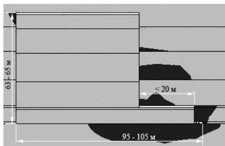
Рис. 5. Распределение зон предельного состояния горных пород при отходе лавы до 95 – 105 м: ■ область действия допустимых напряжений; ■ область предельного состояния
