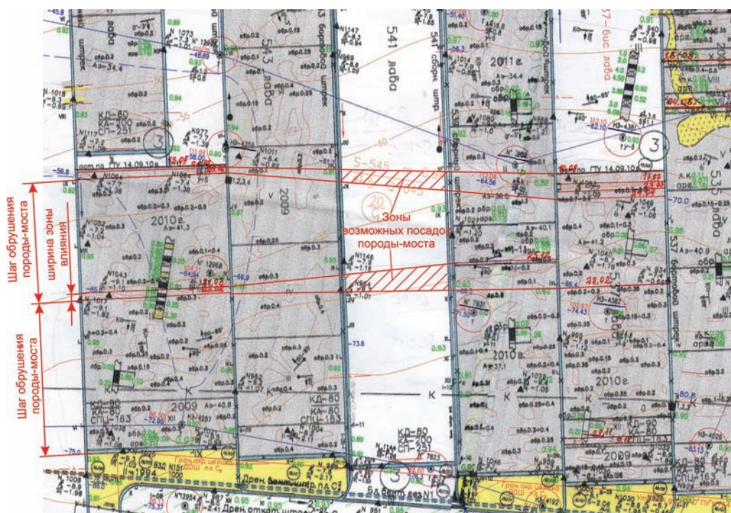
Рис. 1. Выкопировка с плана горных работ по пласту C_5 , с указанием шага обрушения породы-моста, ширины зоны влияния и их возможных посадок
