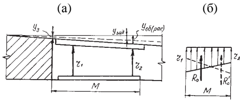
Рис. 4. Схема к расчету сопротивления крепи
