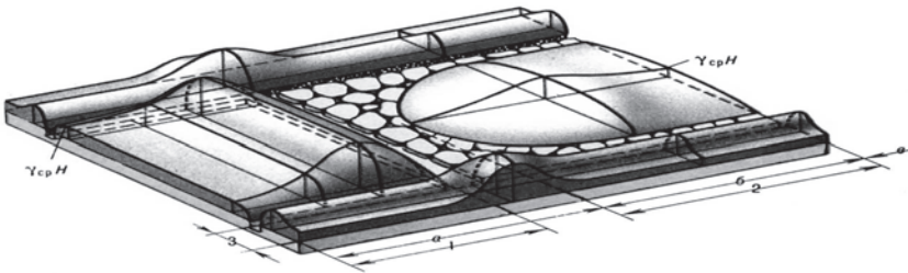
Рис. 2. Гипотетическая картина распределения напряжений вокруг очистной выработки
