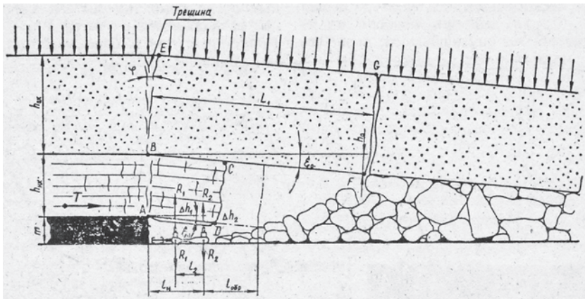
Рис. 3. Схема нагружения крепи в лаве перед осадкой основной кровли
