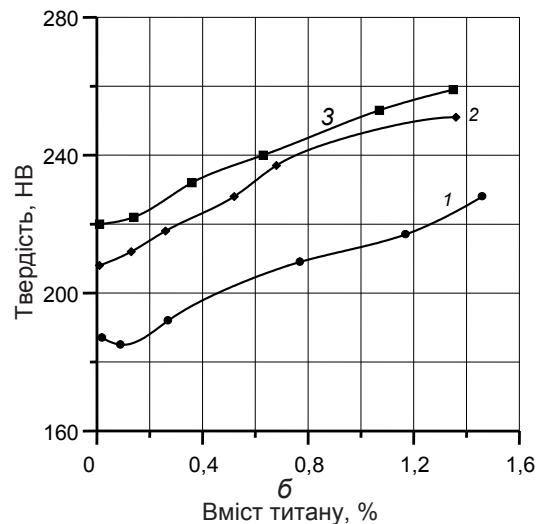
Рис. 4. Вплив титану на міцність (а) та твердість (б) хромоалюмінієвої сталі (%: 30,2 Cr; 1,5 Al) із кількістю вуглецю, %: 1 – 0,08; 2 – 0,4; 3 – 0,8
