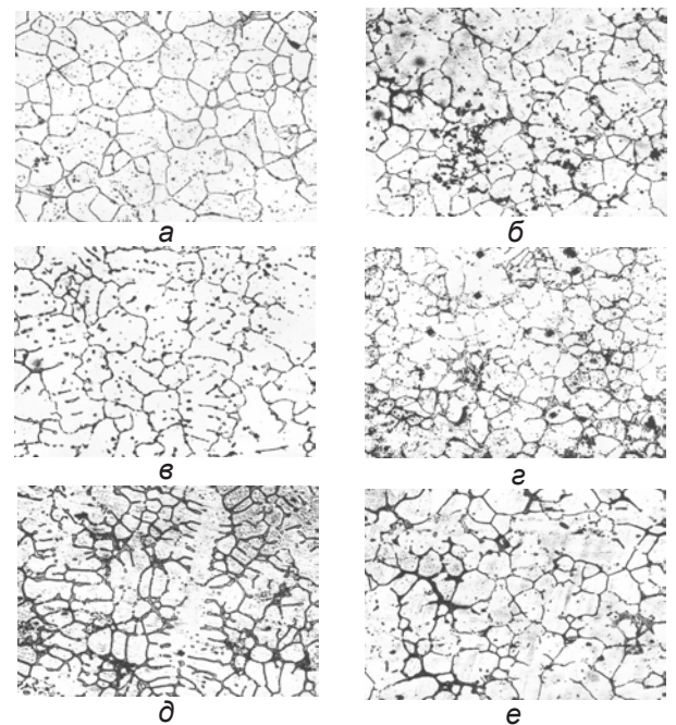
Рис. 3. Мікроструктура хромоалюмінієвої сталі (%: 0,4 С; 30,0 Сr; 1,5 Аl) залежно від вмісту в ній титану, %: без Ті (а); 0,13 (б); 0,26 (в); 0,52 (г); 0,68 (д); 1,36 (е); \times 100
