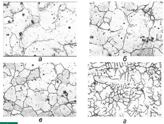
Рис. 2. Мікроструктура хромоалюмінієвої сталі, легованої титаном (%: 0,3 Ті; 30,2 Сr; 1,5 Аl) залежно від вмісту в ній вуглецю, %: 0,10 (а); 0,19 (б); 0,41 (в); 0,79 (г); \times 100
