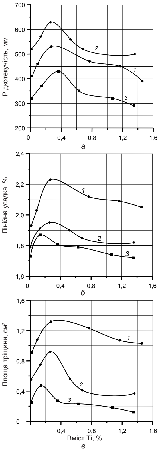
Рис. 1. Вплив титану на рідкотекучість (а), лінійну усадку (б) та тріщинозміцність (в) хромоалюмінієвої сталі, у % (30,2 Сr; 1,5 Аl): 1 – 0,08 С; 2 – 0,4 С; 3 – 0,8 С
