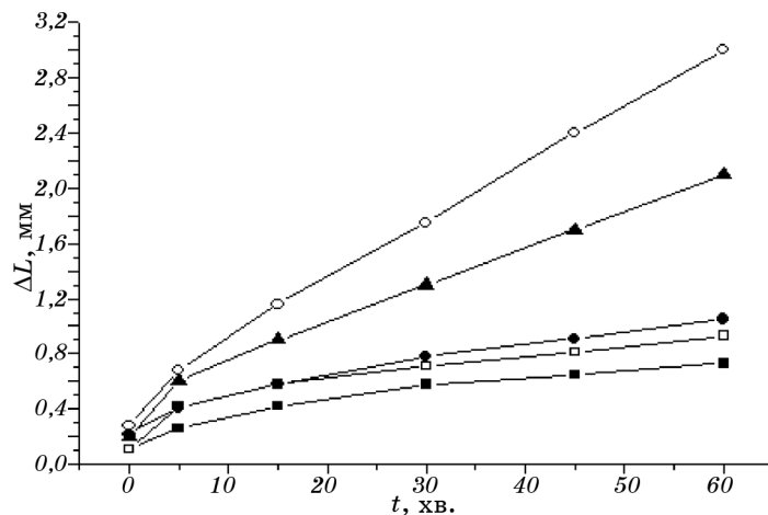
Рис. 5. Криві повзучості сплаву Тi-10-2-3 при різних напруженнях: ■ — 3 МПа, □ — 5 МПа, ● — 15 МПа, ▲ — 20 МПа, ○ — 25 МПа.
