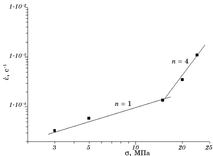
Рис. 6. Залежність швидкості повзучості спеченого сплаву Тi-10-2-3 від напруження.
