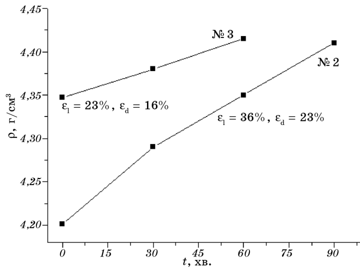
Рис. 9. Залежність густини спеченого сплаву VT6 від часу витримки при повзучості (850°C, \sigma = 30 МПа).
