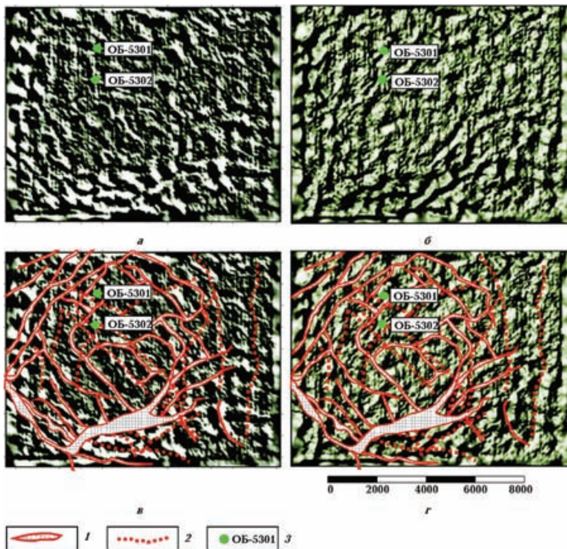
Рис. 5. Теневое изображение нескомпенсированной компоненты гравитационного поля под разными углами освещения (а, б) и закартированные по данным 3D сейсморазведки тектонические нарушения с уточненными и новыми направлениями их распространения по данным линеamentного анализа (в, г): 1 — тектонические нарушения по данным сейсморазведки 3D; 2 — тектонические нарушения, выделенные в результате сейсмогравитационного моделирования; 3 — поисково-картировочные скважины, пробуренные в пределах Оболонской площади.
